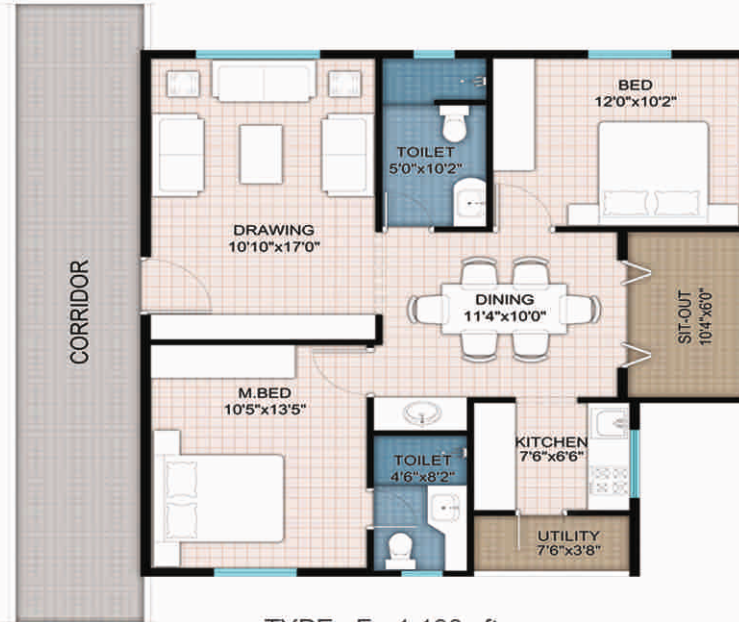
TYPE : F - 1,130 sft.
